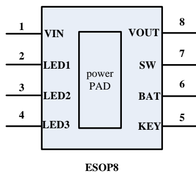
图 2 IP5305/IP5305T 引脚图
