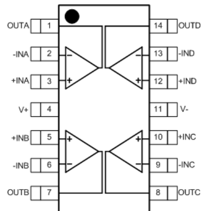
SOIC-14/TSSOP-14
