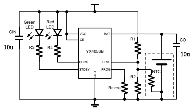
图 1. 典型应用电路
